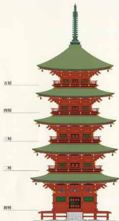
大石寺五重塔正面図 高さ 34.3m
